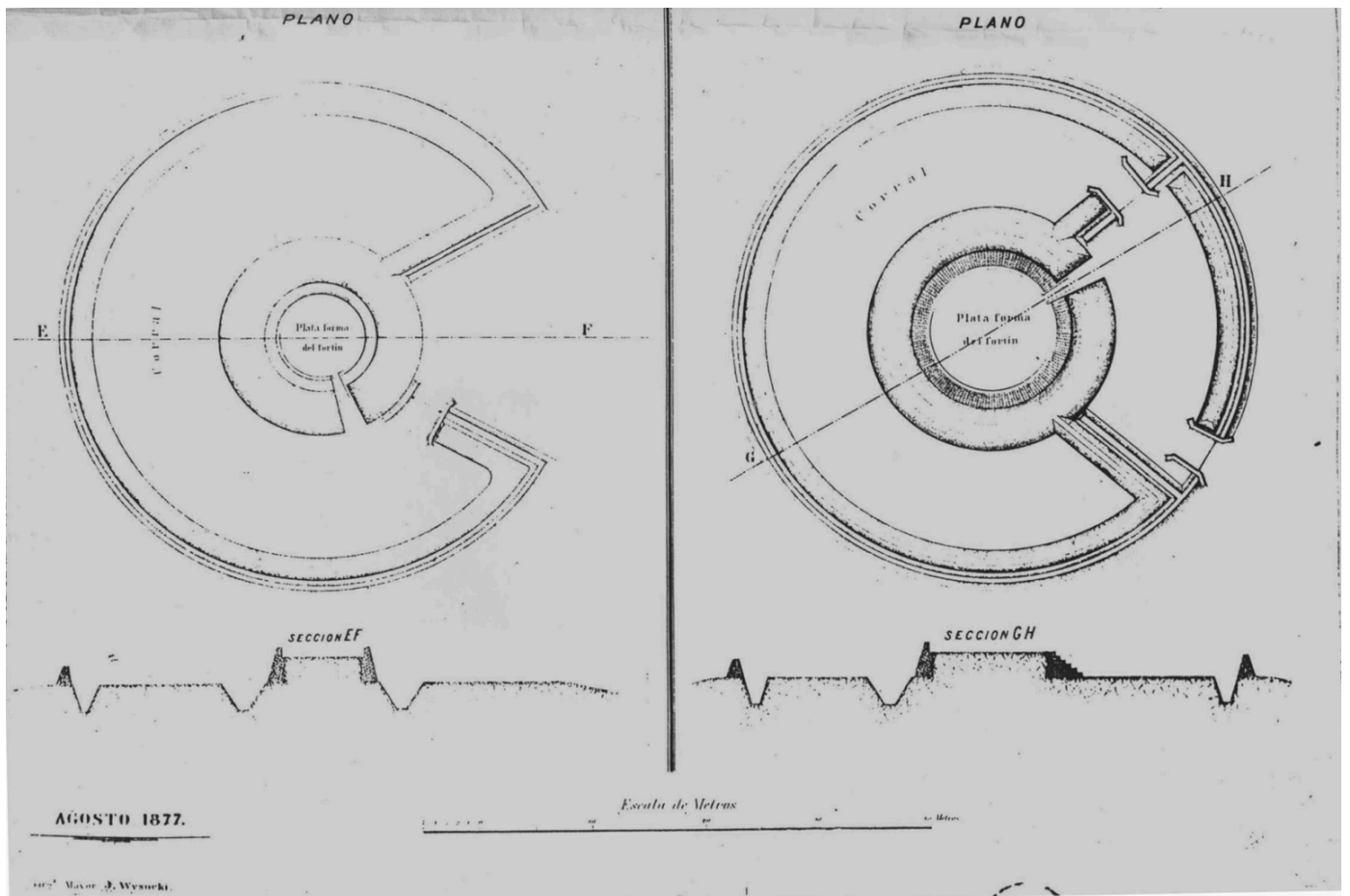
Plano de construcción de un fortín, 1877. Fuente: Archivo General de la Nación.
